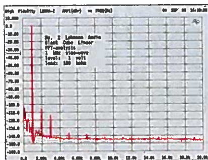
Forforstærkerens linearitet er ganske overbevisende. THD+N aflæses til 0,0012% ved 1 volt ud. Det er oven i købet den 2. harmoniske der dominerer.
