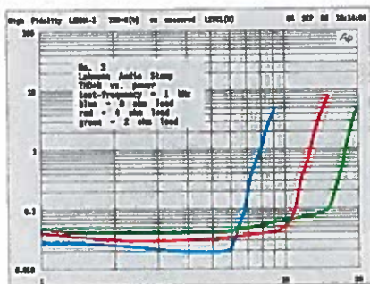
Stamp effektforstærkeren er uden tvivl en af de effektmæssigt mindste forstærkere vi nogensinde har målt på: 6/10/15 W i 8/4/2 ohm.
