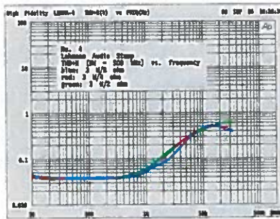
Ved 3 W ud i 8/4/2 ohm er forvrængningen (THD+N) jævnt tiltagende over 1 kHz, men forløbene er nærmest helt uafhængige af belastningsimpedansen.
