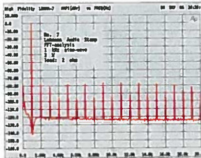
Når man giver den lille forstærker til opgave at afgive 3 W i kun 2 ohm stiger THD+N til 0,050%, men spektret er stort set det samme som ved 4 ohms belastning.
