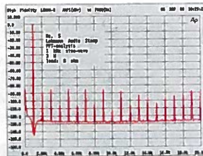
Ved 3 W i 8 ohm aflæses THD+N til 0,022%. Som det tydeligt fremgår er hele det hørbare spektrum dækket ind af harmoniske, der overvejende er af ulige orden.
