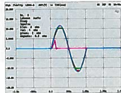
Impulsmæssigt kan den lille Stamp levere lidt over 10 Vpeak i både 8, 4 og 2 ohm (= 1,5/2,9/5,2 A), men de 0,6 ohm bryder den sig bestemt ikke om.
