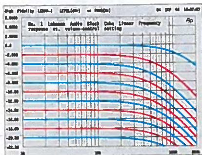
Med volumenkontrollen i max. er den lille forforstærkers båndbredde (-3 dB) 145 kHz, men ved -6 dB er den reduceret til ca. 60 kHz.
